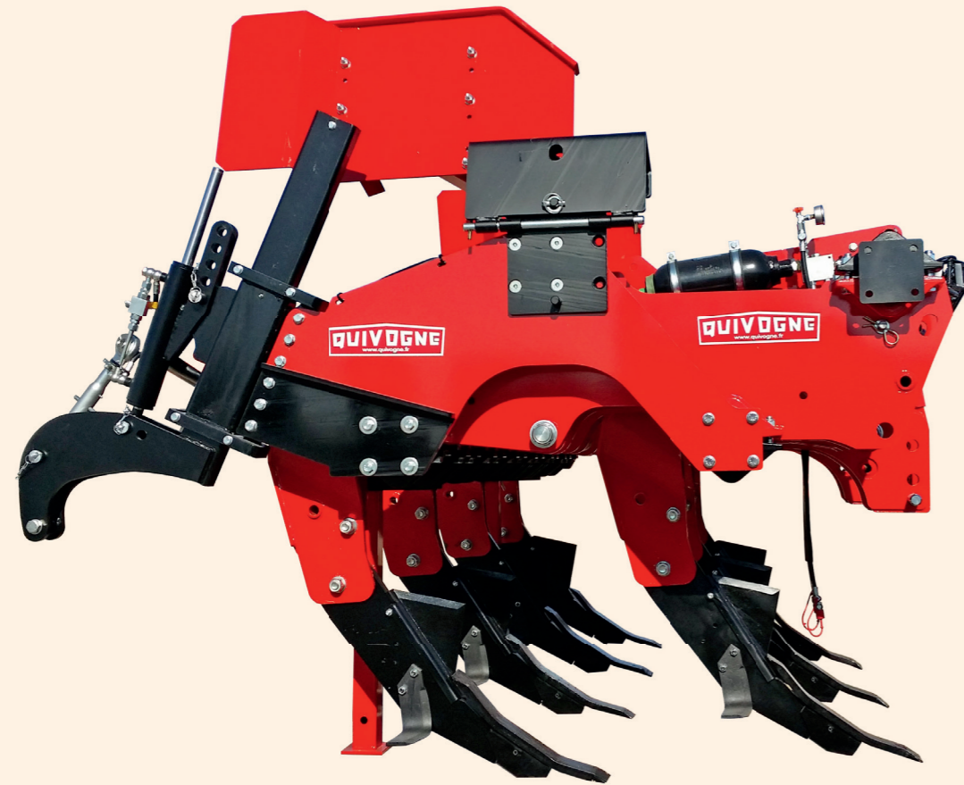
Kép: SSSDR NON-STOP 7/300 oldalsó terelőlemezrel, hidroakkumulátorral és hidraulikus hengerállítással (henger nélkül)
