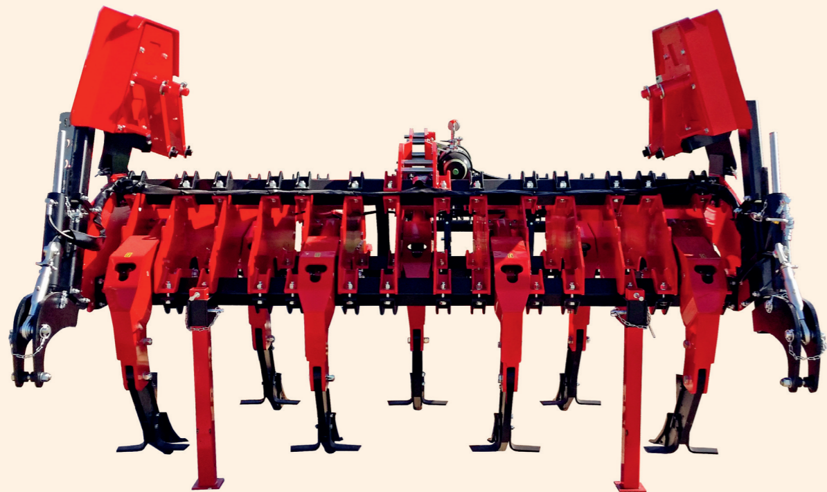
Kép: SSDR NON-STOP 7/300 oldalsó terelőlemezzel, hidraulikus állítás (henger nélkül), támasztólábbal és mélységmutatóval
